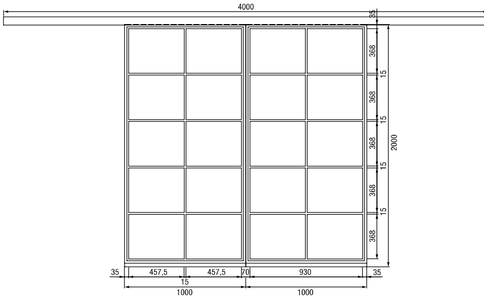
2-flügelige Stahl-Lofttür
