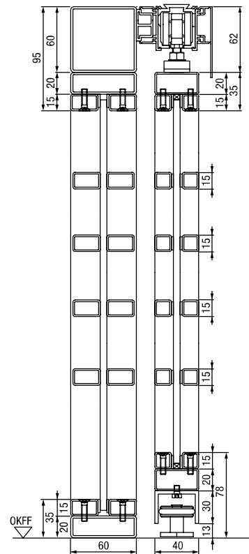
Vertikalschnitt 2-flügelige Stahl-Lofttür mit Seitenteil
