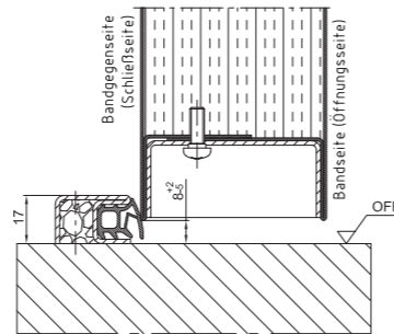
RS1/RS1V absenkbare Bodendichtung
