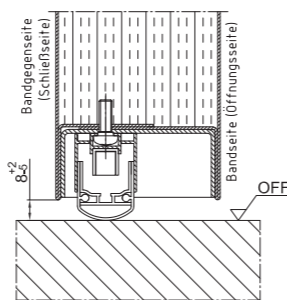
RS1/RS1V absenkbare Bodendichtung
