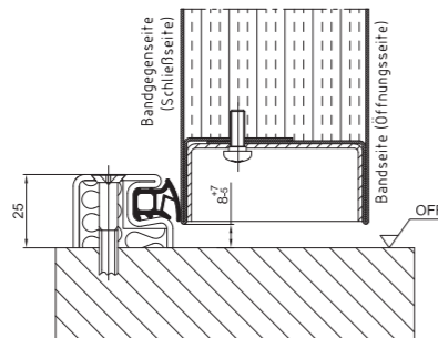
C2 Schwelle mit unterem Anschlag und Dichtung bei Zarge mit Bodeneinstand 2)
