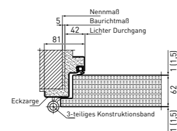
Horizontalschnitt 2-flgl.
