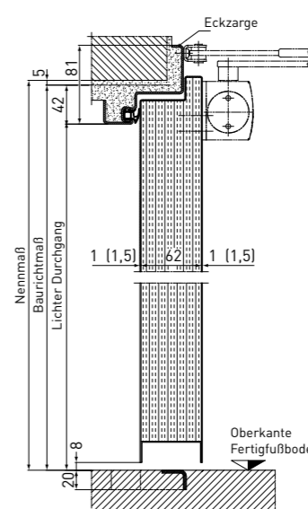
Vertikalschnitt
