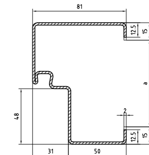
Montage in der Laibung
