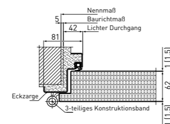
Horizontalschnitt 2-flgl.
