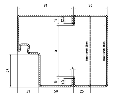
Montage in der Laibung
