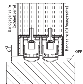
2xRS1 doppelt absenkbare Bodendichtung 2)
