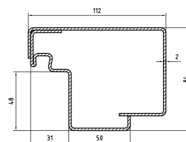
Montage in der Laibung
