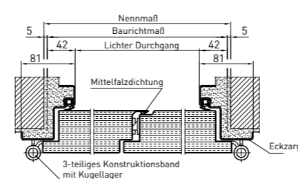
Horizontalschnitt 2-flgl.
