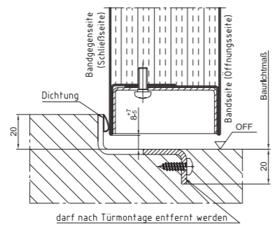
RS2 Dichtungsschwelle/Höckerschwelle 1)2)
