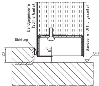
2xRS1 doppelt absenkbare Bodendichtung 2)
