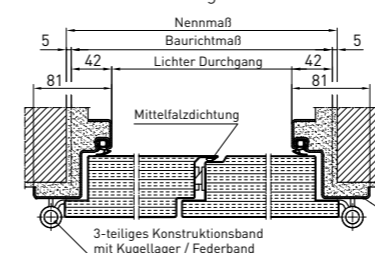
Horizontalschnitt 2-flgl.
