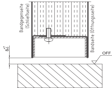
B2 Schwelle für kleine Türen bis BRM-Höhe 1749 mm und Türen ab BRM-Höhe 1750 mm 4-seitig umlaufender Rahmen (Zarge 4-seitig umlaufend) 4)
