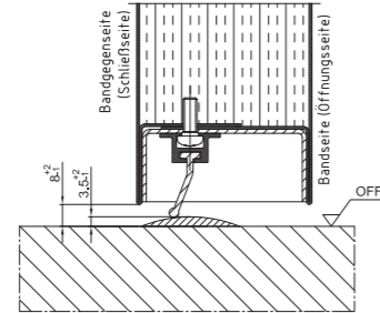
RS2 Dichtungsschwelle/Höckerschwelle 1)2)
