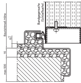
C2 Schwelle mit unterem Anschlag und Dichtung 2)
