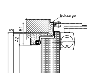
Vertikalschnitt
