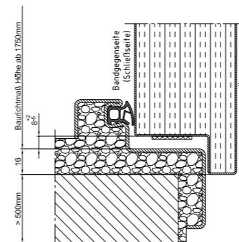
B1 Schwelle für Türen mit 4-seitig umlaufenden Rahmen (Türblatt und Zarge 4-seitig umlaufend)
