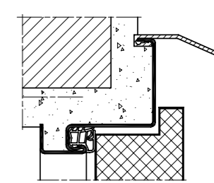
erforderlich bei Außeneinsatz und Schlagregen (nur bei MZ und EI 2 30/60/90 in der Außenanwendung möglich)
