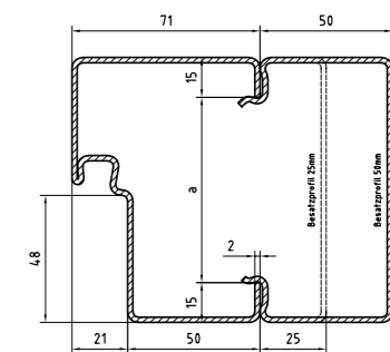
Montage in der Laibung
