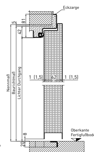
Vertikalschnitt
