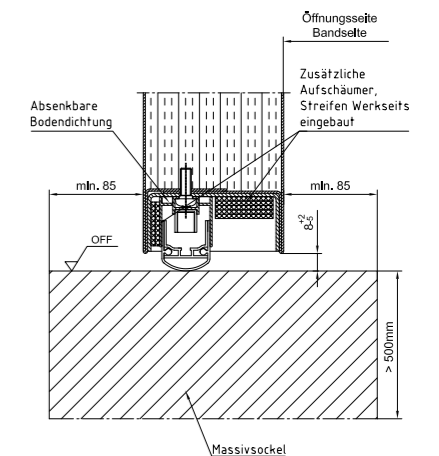
B1 Schwelle für Wandklappen mit 4-seitig umlaufenden Rahmen (Türblatt und Zarge 4-seitig umlaufend)
